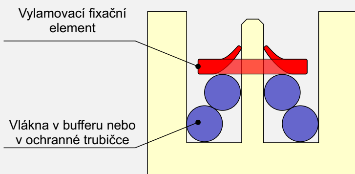
Detail zásobníku rezerv vláken
