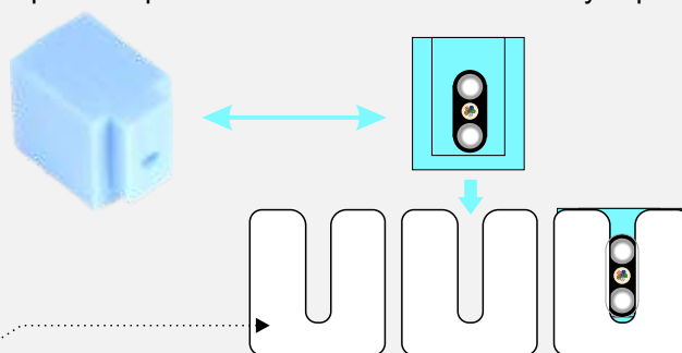
Zářezový fixační člen pro plochý kabel
