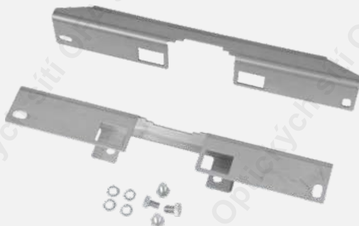
Držák spojky BPEO S2,3 na zeď/sloup
