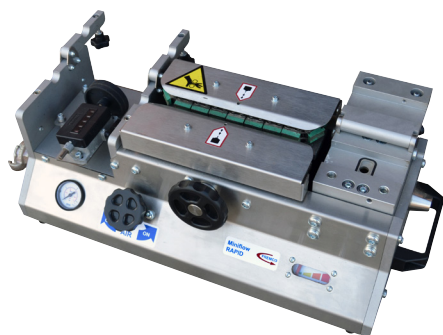
Základní konfigurace včetně řetězů.
