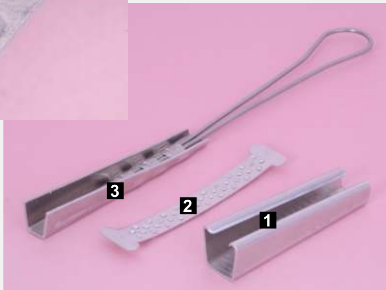
Obr. 1- rozložená kotva
